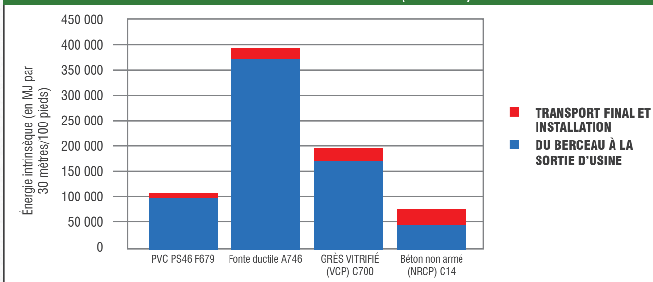
FIGURE 12.8: ÉNERGIE INTRINSÈQUE TOTALE SUR 100 ANS DE TUYAUX EN PVC ÉQUIVALENTS PS46 F679 À PAROI PLEINE DE 600 MM (24 POUCES)
