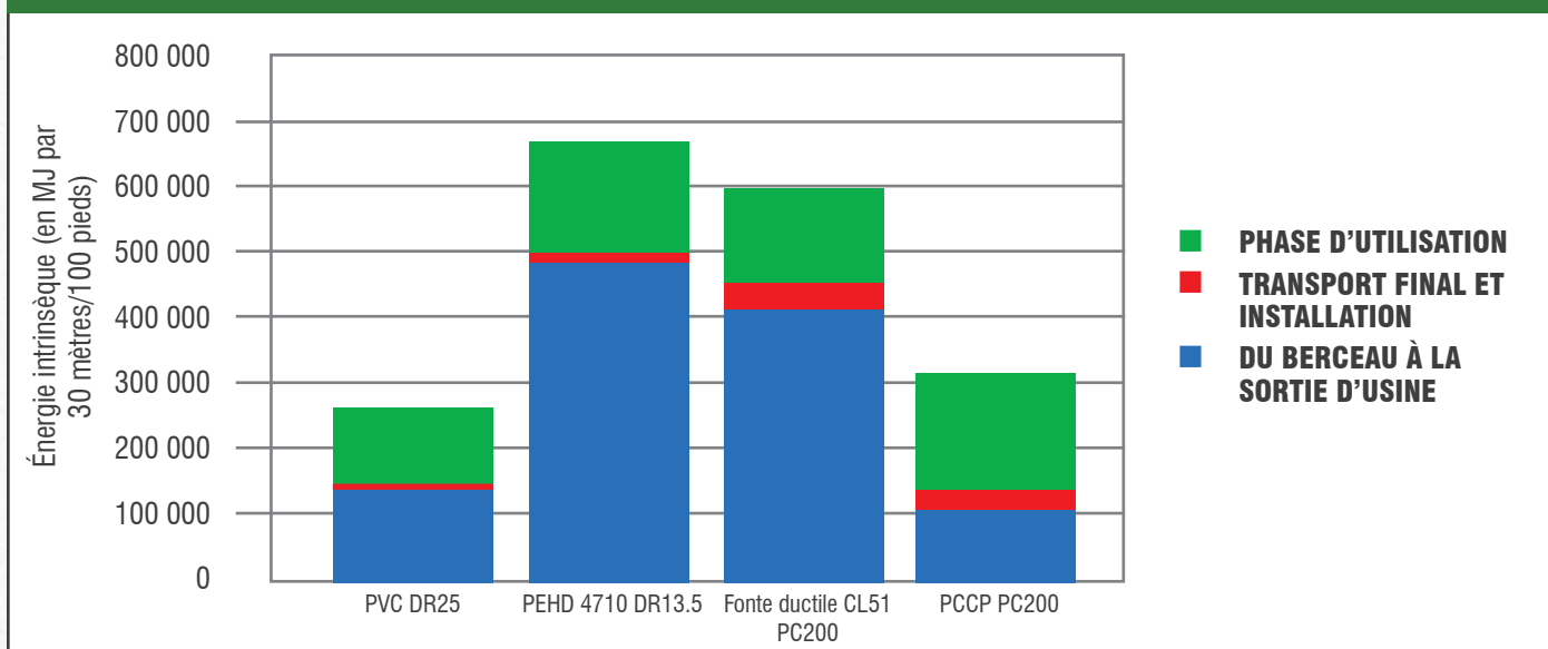
FIGURE 12.3: ÉNERGIE INTRINSÈQUE TOTALE SUR 100 ANS DE TUYAUX EN PVC ÉQUIVALENTS DR25 DE 600 MM (24 POUCES)
