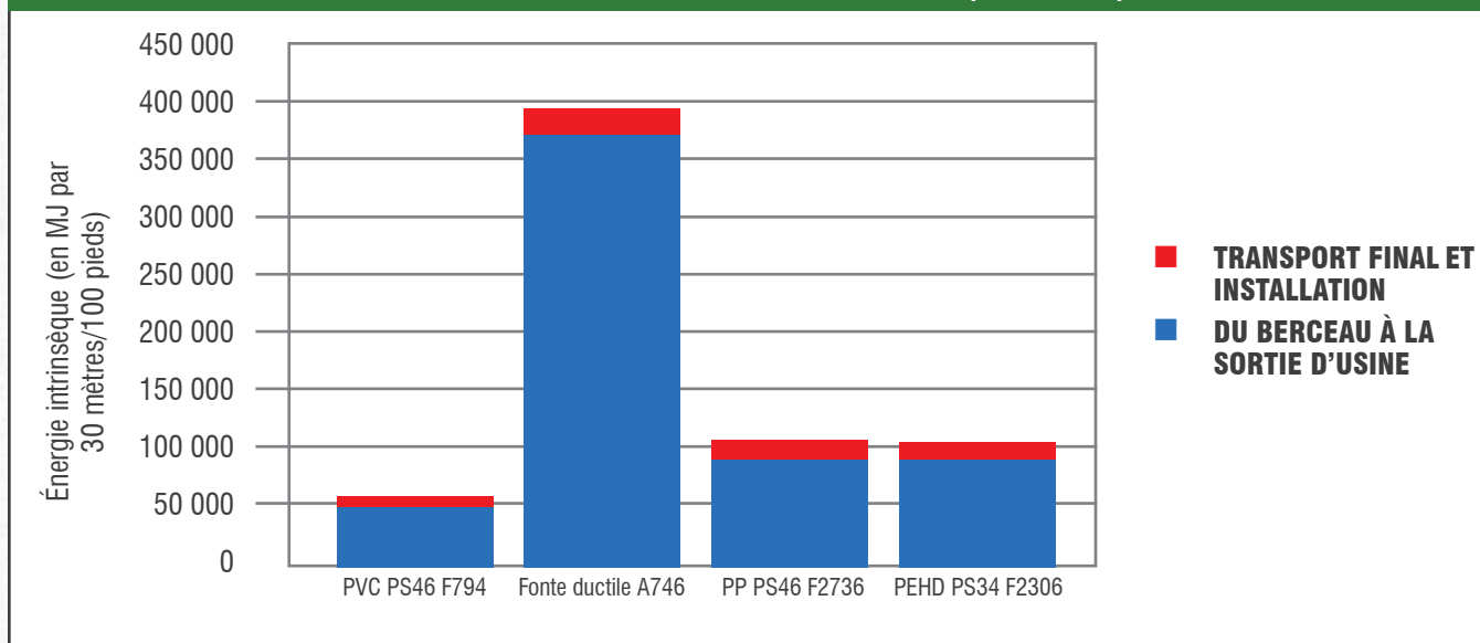
FIGURE 12.7: ÉNERGIE INTRINSÈQUE TOTALE SUR 100 ANS DE TUYAUX EN PVC ÉQUIVALENTS PS46 F794 À PAROI NERVURÉE DE 600 MM (24 POUCES)
