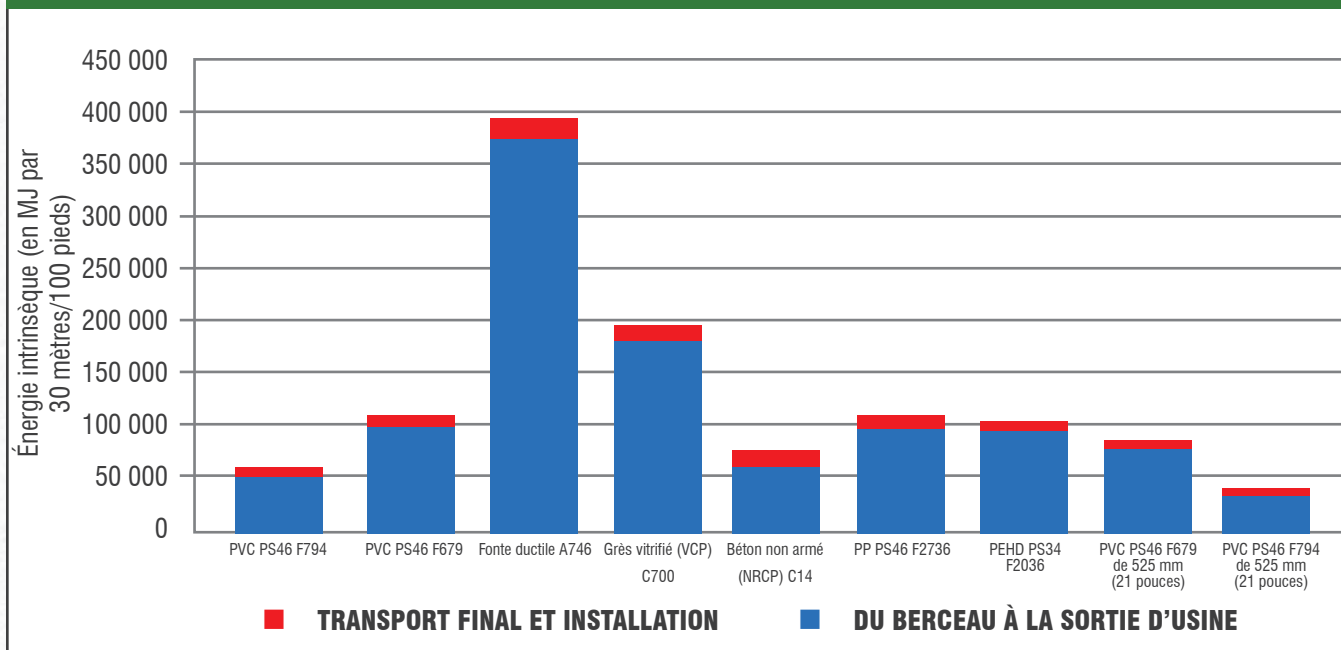
FIGURE 12.9: ÉNERGIE INTRINSÈQUE TOTALE SUR 100 ANS DE TUYAUX EN PVC ÉQUIVALENTS PS46 À PAROI PLEINE OU PAROI NERVURÉE DE 600 MM (24 POUCES)
