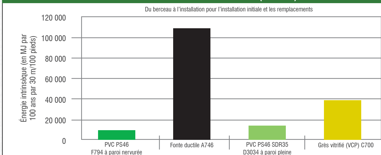
FIGURE A.9 : ÉNERGIE INTRINSÈQUE TOTALE SUR 100 ANS DE PRODUITS DE TUYAUX À ÉCOULEMENT PAR GRAVITÉ DE 200 MM (8 POUCES)
