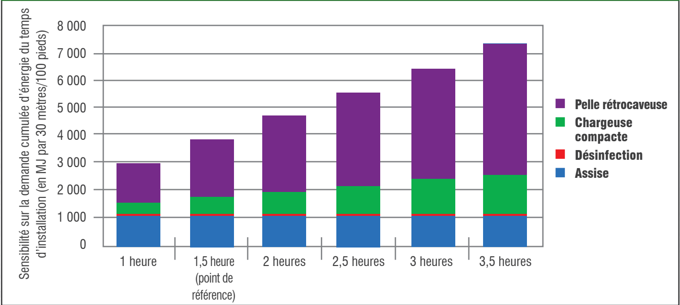
FIGURE 6.2: ANALYSE DE SENSIBILITÉ DES TEMPS D'INSTALLATION DE TUYAUX SOUS PRESSION DE 200MM (8 POUCES) DE DIAMÈTRE DE 30 M (100 PIEDS) DE LONG (DEMANDE CUMULÉE D'ÉNERGIE, EN MJ PAR 30 MÈTRES/100 PIEDS)
