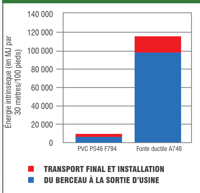
FIGURE 12.5 : ÉNERGIE INTRINSÈQUE TOTALE SUR 100 ANS DE TUYAUX EN PVC ÉQUIVALENTS PS46 F794 À PAROI NERVURÉE DE 200 MM (8 POUCES)
