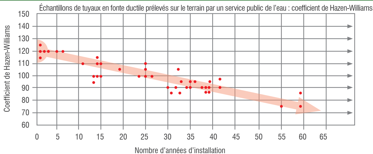
FIGURE 8.5: ÉCHANTILLONS PRÉLEVÉS SUR LE TERRAIN MONTRANT LA BAISSSE DU FACTEUR « C » AU FIL DU TEMPS POUR DES TUYAUX EN FONTE DUCTILE
