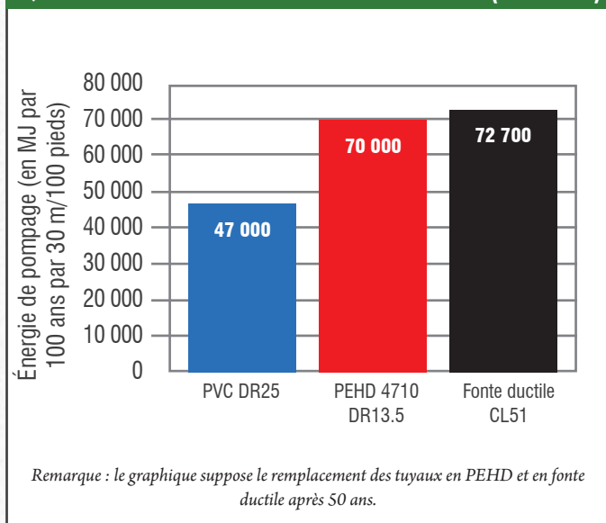
FIGURE A.17 : ÉNERGIE DE POMPAGE SUR 100 ANS DE TUYAUX ÉQUIVALENTS AUX TUYAUX PVC DR25 DE 200 MM (8 POUCES)
