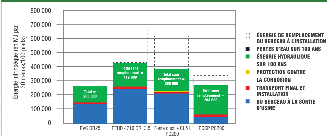
FIGURE 12.4 : ÉNERGIE INTRINSÈQUE TOTALE SUR 100 ANS DE TUYAUX EN PVC ÉQUIVALENTS DR25 DE 600 MM (24 POUCES) (ÉNERGIE HYDRAULIQUE SANS REMPLACEMENT)
