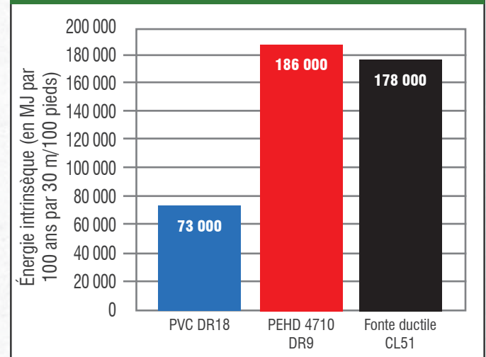
FIGURE 10.5 : ÉNERGIE INTRINSÈQUE TOTALE SUR 100 ANS DE TUYAUX ÉQUIVALENTS AUX TUYAUX DR18 DE 200 MM (8 POUCHES)
