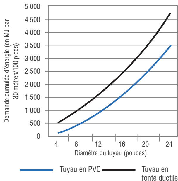
FIGURE 6.1 : DEMANDE CUMULÉE D'ÉNERGIE POUR LE TRANSPORT
