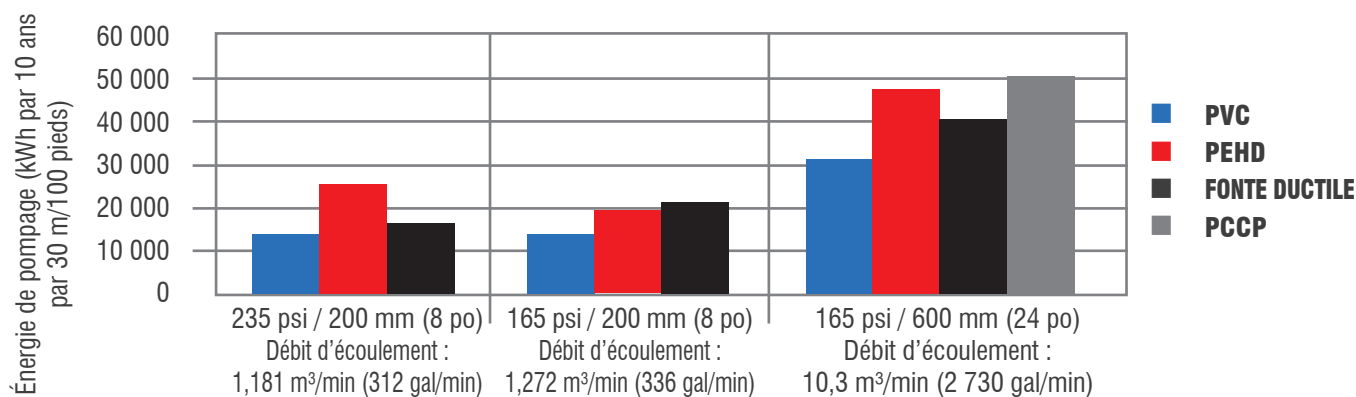
FIGURE A.3 : CONSOMMATION ÉNERGÉTIQUE DE POMPAGE SUR 100 ANS, POUR 30 MÈTRES (100 PIEDS) DE TUYAU
