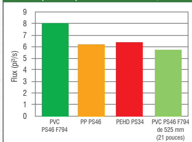
FIGURE A.11 : COMPARAISON DES FLUX D'ÉCOULEMENT DANS DES TUYAUX À ÉCOULEMENT PAR GRAVITÉ EN PVC À PAROI NERVURÉE DE 600 MM (24 POUCES) À ANGLES D'INCLINAISON ÉQUIVALENTS
