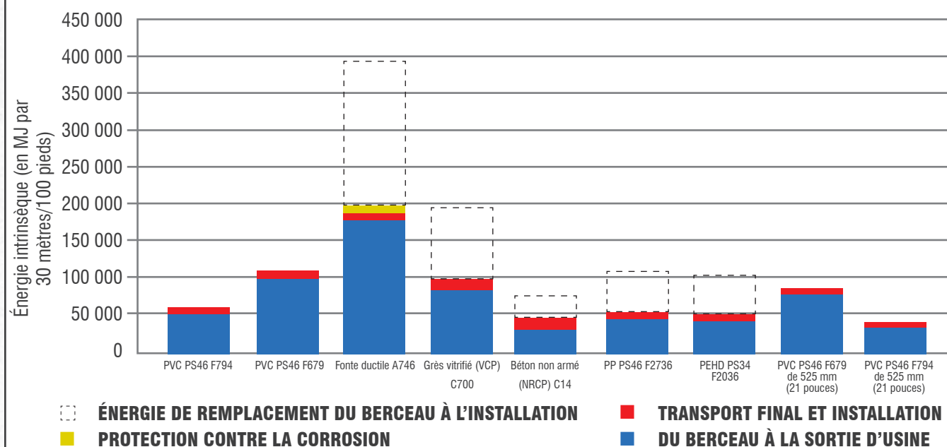
FIGURE 12.10: ÉNERGIE INTRINSÈQUE TOTALE SUR 100 ANS DE TUYAUX EN PVC ÉQUIVALENTS PS46 À PAROI PLEINE OU PAROI NERVURÉE DE 600 MM (24 POUCES)
