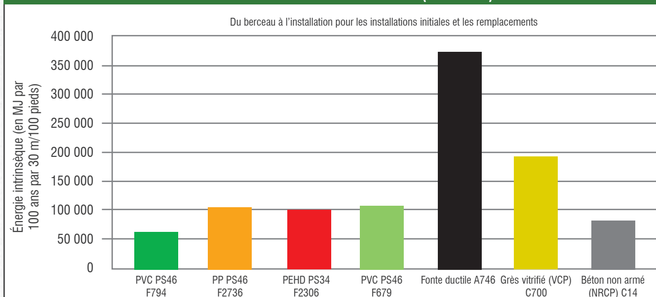
FIGURE A.8 : ÉNERGIE INTRINSÈQUE TOTALE SUR 100 ANS DE PRODUITS DE TUYAUX À ÉCOULEMENT PAR GRAVITÉ DE 600 MM (24 POUCES)
