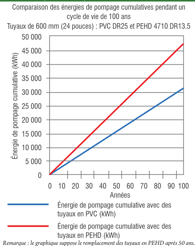
FIGURE 9.6 : COMPARAISON DES ÉNERGIES DE POMPAGE CUMULATIVES SUR 100 ANS DE TUYAUX DE 600 MM (24 POUCES) EN PVC ET EN PEHD
