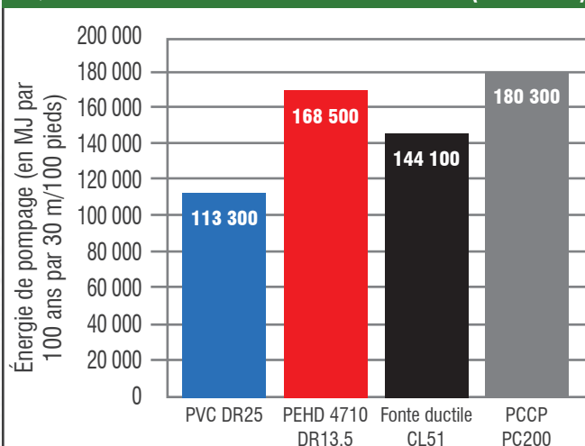
FIGURE A.18 : ÉNERGIE DE POMPAGE SUR 100 ANS DE TUYAUX ÉQUIVALENTS AUX TUYAUX PVC DR25 DE 600 MM (24 POUCES)
