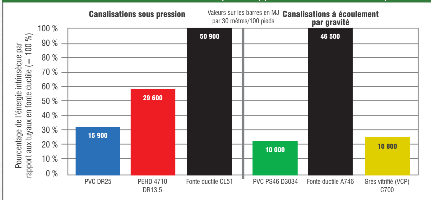
FIGURE A.14 : COMPARAISON DES VALEURS DE L'ÉNERGIE INTRINSÈQUE DE LA CRÉATION À LA SORTIE D'USINE POUR DES TUYAUX EN PVC ÉQUIVALENTS DR25 DE 200 MM (8 POUCES) (EN MJ PAR 30 MÈTRES/100 PIEDS)
