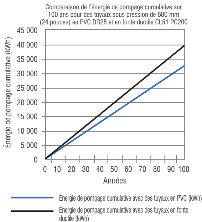
FIGURE 9.2 : COMPARAISON DES ÉNERGIES DE POMPAGE CUMULATIVES SUR 100 ANS DE TUYAUX DE 600 MM (24 POUCES) EN PVC ET EN FONTE DUCTILE
