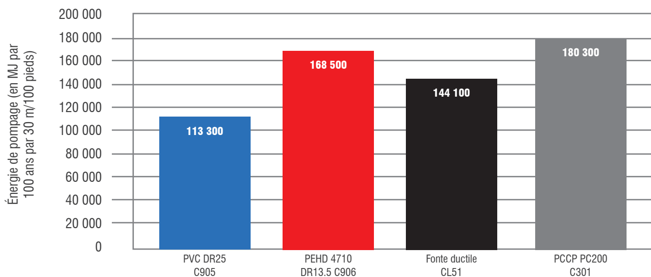
FIGURE A.19 : ÉNERGIE DE POMPAGE SUR 100 ANS DE TUYAUX ÉQUIVALENTS AUX TUYAUX PVC DR25 DE 600 MM (24 POUCES)
