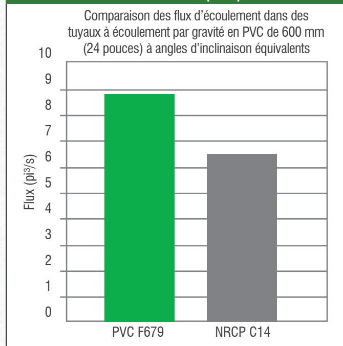
FIGURE 9.4 : COMPARAISON DES FLUX D'ÉCOULEMENT DANS DES TUYAUX DE 600 MM (24 POUCES), EN PVC À PAROI PLEINE ET EN BÉTON NON ARMÉ (NRCP)
