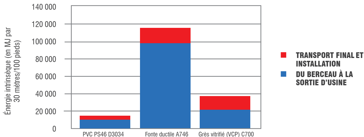
FIGURE 12.6 : ÉNERGIE INTRINSÈQUE TOTALE SUR 100 ANS DE TUYAUX EN PVC ÉQUIVALENTS PS46 D3034 À PAROI PLEINE DE 200 MM (8 POUCES)
