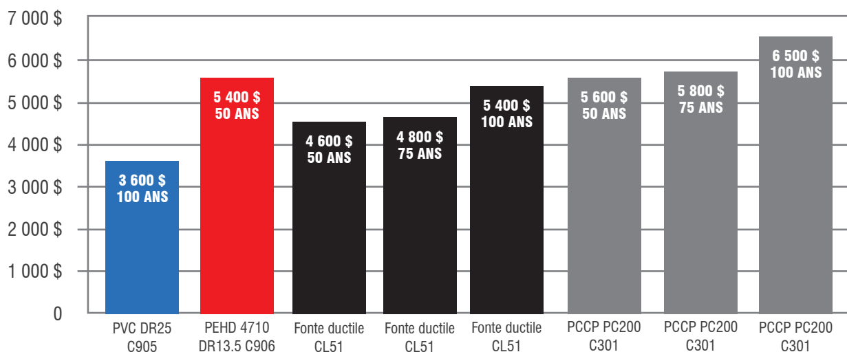
FIGURE A.22 : COÛTS ÉNERGÉTIQUES DE POMPAGE SUR 100 ANS POUR DES TUYAUX EN PVC ÉQUIVALENTS DR25 DE 600 MM (24 POUCES) POUR DIFFÉRENTES VALEURS DE LA DURÉE DE VIE UTILE ($ PAR 30 MÈTRES SUR 100 ANS)
