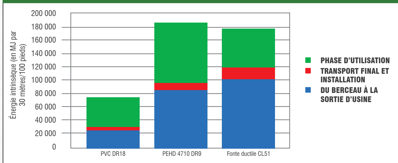
FIGURE 12.1: ÉNERGIE INTRINSÈQUE TOTALE SUR 100 ANS DE TUYAUX EN PVC ÉQUIVALENTS DR18 DE 200 MM (8 POUCES)
