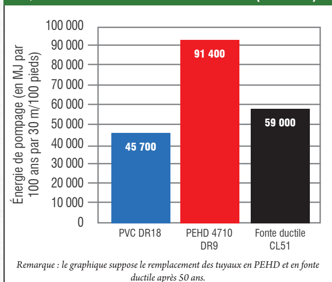
FIGURE A.16 : ÉNERGIE DE POMPAGE SUR 100 ANS DE TUYAUX ÉQUIVALENTS AUX TUYAUX DR18 DE 200 MM (8 POUCES)
