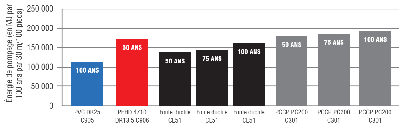
FIGURE A.20 : CONSOMMATION ÉNERGÉTIQUE DE POMPAGE SUR 100 ANS POUR DES TUYAUX EN PVC ÉQUIVALENTS DR25 DE 600 MM (24 POUCES) POUR DIFFÉRENTES VALEURS DE LA DURÉE DE VIE UTILE
