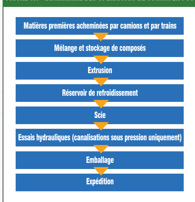
FIGURE 5.3 : DIAGRAMME DES OPÉRATIONS DE TUYAUX EN PVC
